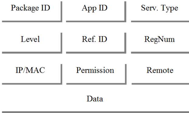
Fig. 3. SSIL Frame
